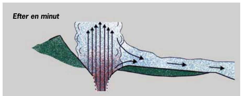
Efter en minuts utbrott börjar den 930 grader heta magman spruta genom vulkanens krater rakt upp i luften från sin källa 10 km under jorden. Sedan kollapsar magman och bildar en pyroklastisk ström som väller nerför berget i sex timmar. Sedan 1986, när berget stabiliserats efter utbrottet, är Mount St. Helens bara 2549 meter högt, 400 m lägre än före utbrottet.
