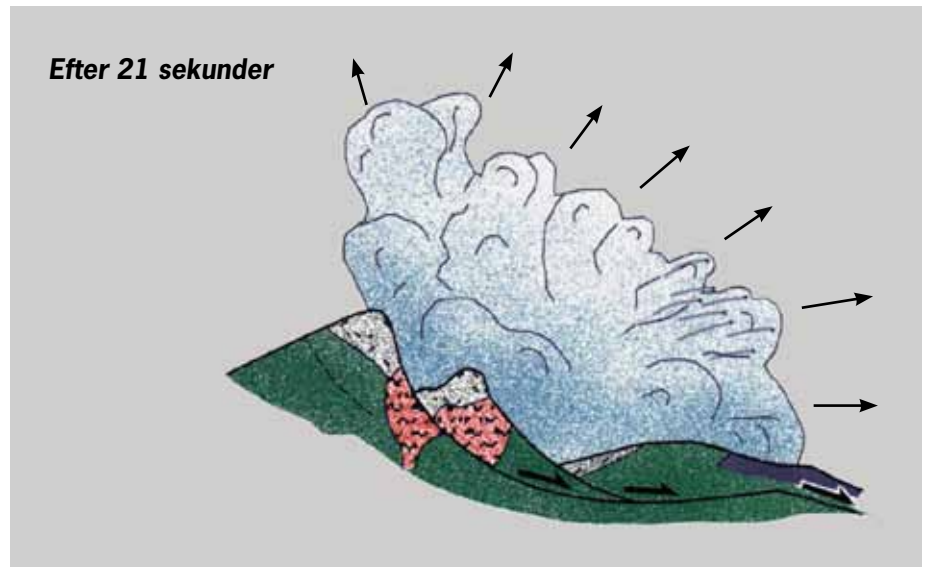
14 sekunder efter utbrottets början brister bergets norra sida och ger upphov till tre stora jordskred. Överhettat vatten inuti vulkanen sprutar ut. Sten och klippblock far iväg som projektiler mot norr. 7 sekunder senare rutschar 2,5 miljarder kubikmeter sten och lera iväg nerför berget till dalen i norr.
