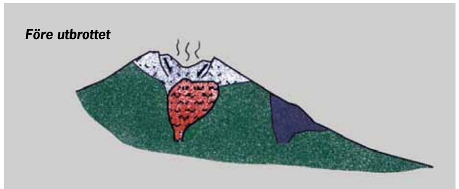
Den 18 maj, 1980 före utbrottet. Magma har trängt upp mot kraterns yta och skapat en bula på bergets norra (högra) sida. Berget var 2950 m högt före vulkanutbrottet.
